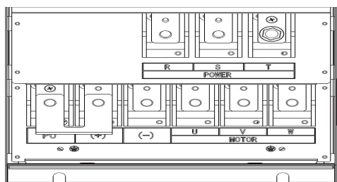
(g) 主回路功率端子 (132-185kW)
