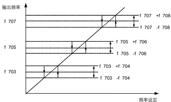
图 6.34 跳跃频率参数设置示意
