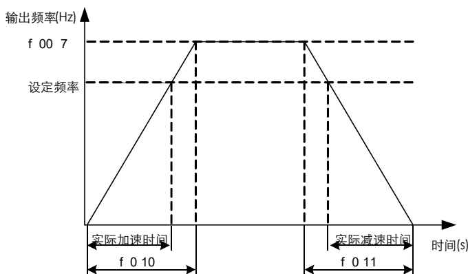
图 6.3 加速时间和减速时间定义
