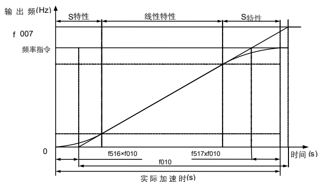
图 6.28 S 型曲线 1
