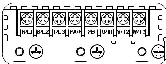
(a) 主回路功率端子 (11kW (含) 以下)
