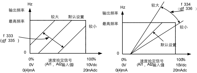
图 6.12 模拟输入校准
