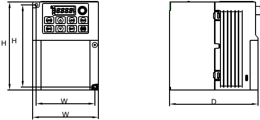
图 3.2 外形及安装尺寸图 (三相 11kW (含) 以下)
