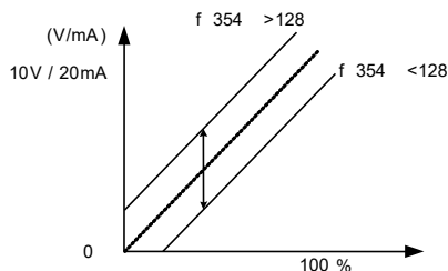
图 6.20 模拟输出曲线与 f354 关系
