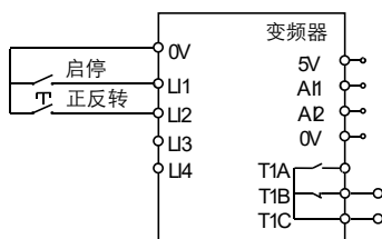
图 5.13 2 线控制模式 2-按钮开关正反转控制接线示意图
