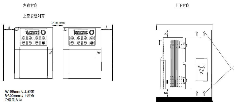
图 4.3 多台左右安装间距要求
