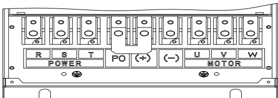
(d) 主回路功率端子 (45kW)
