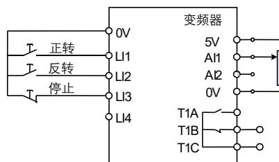
图 5.8 3 线控制 (负逻辑) 接线示意图
