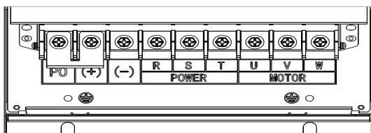
(e) 主回路功率端子 (55kW)
