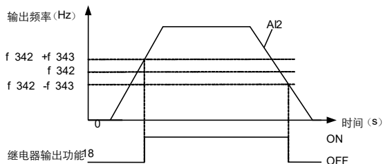
图 6.16 继电器输出-A11 输入检出示意图
