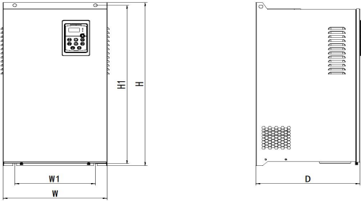
图 3.3 外形及安装尺寸示意图（三相 15KW-315kW）
