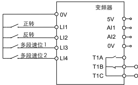
图 5.10 多段速控制接线示意图
