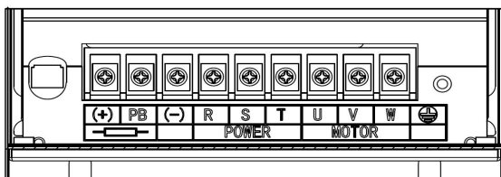
(b) 主回路功率端子 (15-22kW)
