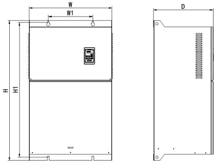
图 3.4 外形及安装尺寸示意图（三相 355kW-500kW）
