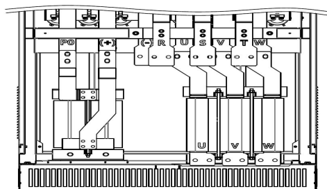
(k) 主回路功率端子 (560-800kW) 壁挂式
