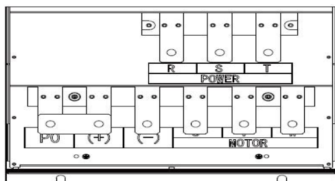
(h) 主回路功率端子 (200-220kW) 壁挂式
