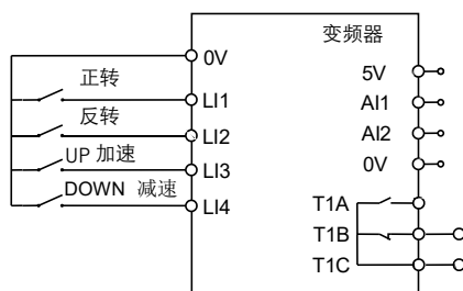
图 5.9 UP/DOWN 加减速接线示意图
