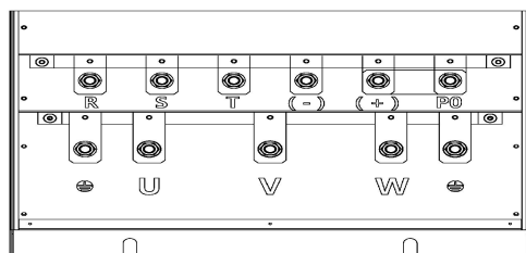
(j) 主回路功率端子 (355-500kW) 壁挂式
