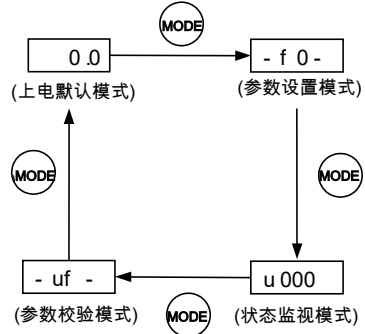
图 5.2 变频器模式切换示意图
