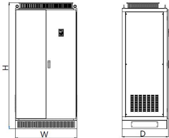
图 3.5 外形及安装尺寸示意图（三相 560kW-800kW）
