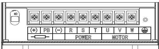
(c) 主回路功率端子 (30-37kW)
