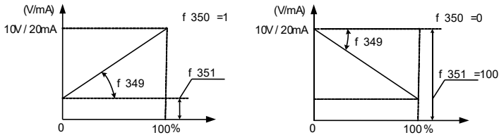
图 6.18 参数 f349, f350 和 f351 设置示意图
