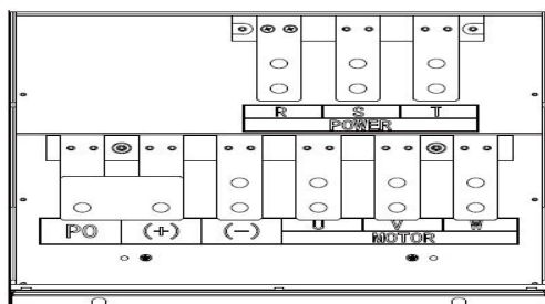
(i) 主回路功率端子 (250-315kW)
