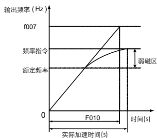
图 6.29 S 型曲线 2
