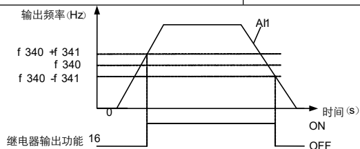
图 6.15 继电器输出-A11 输入检出示意图
