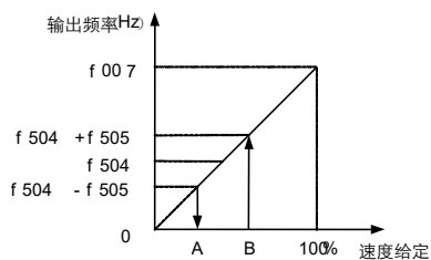
图 6.26 运行起始频率
