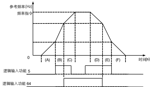
图 6.32 通过逻辑输入切换加减速曲线
