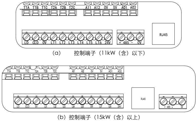
图 4.8 控制端子结构示意图
