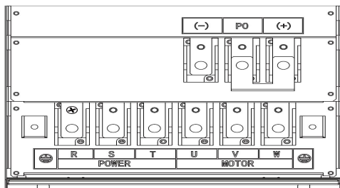
(f) 主回路功率端子 (75-110kW)
